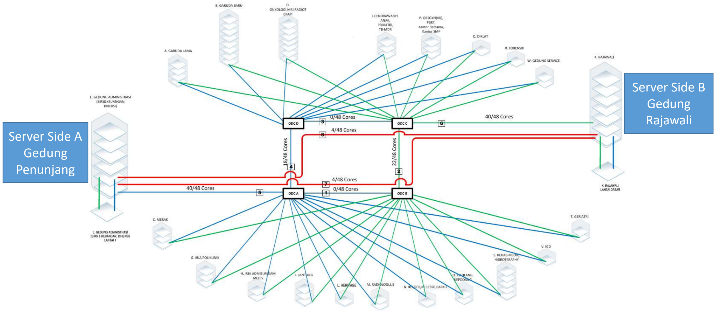
Gambar Desain Topologi Distribusi FO Seluruh Gedung RSDK
